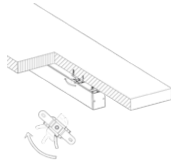
Deckenhalterung 2 Stk Art.Nr. 457060 9,50 €
